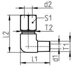
B: 90° Winkel / 90° angle
