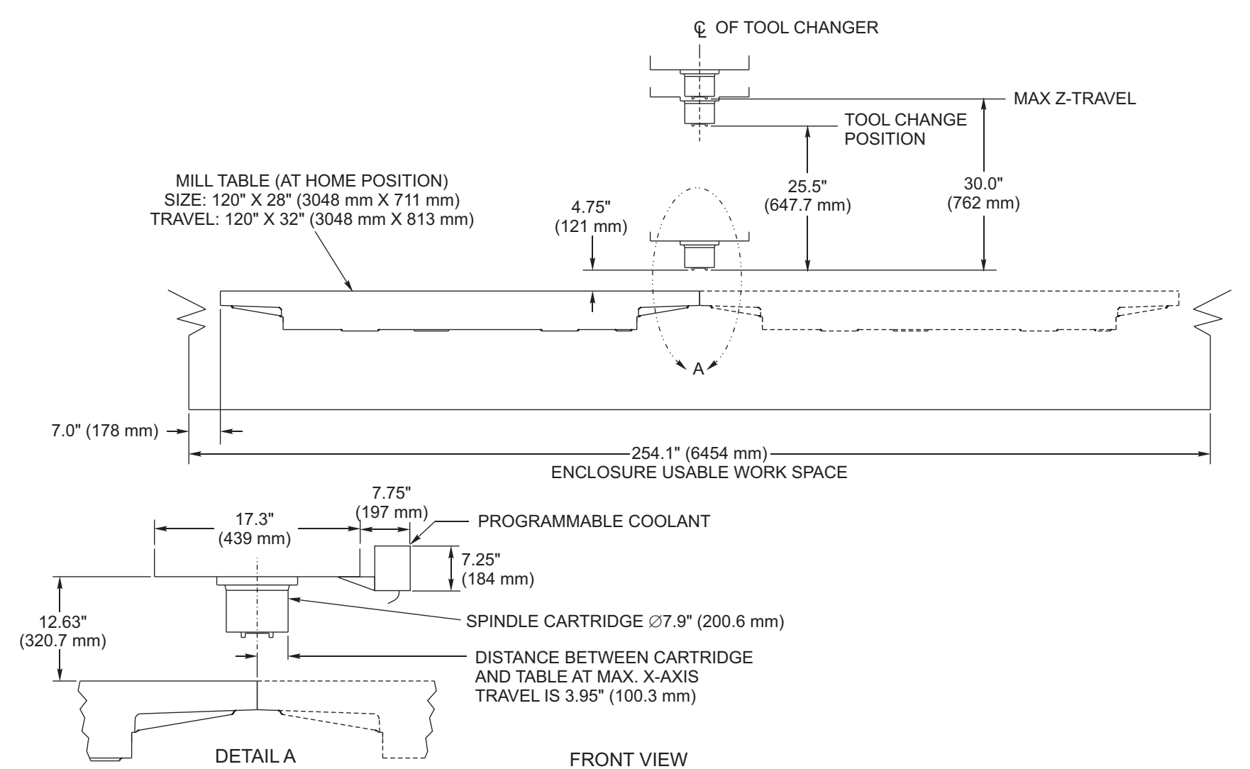
VF11-50 Table Dimensions
