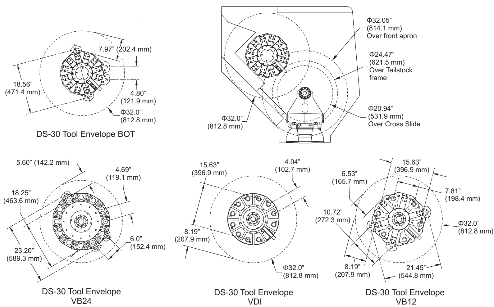
DS-30 Tool Envelopes
